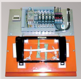
■ 部品欠品検査治具
