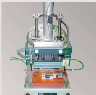
■ 熱加締め治具
