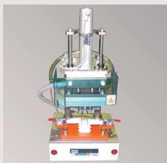
■ ゲートカット治具
